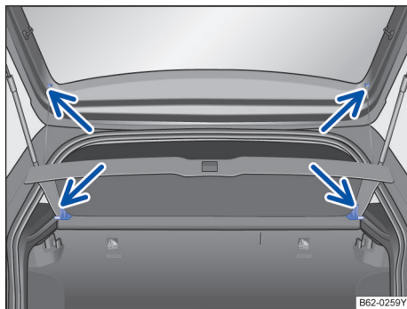
图 122 拆卸和安装行李厢盖板
