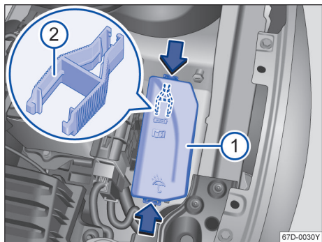
图 133 发动机舱内：保险丝盒盖板
