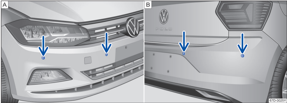
图 105 前后保险杠：驻车距离警报系统超声波传感器
