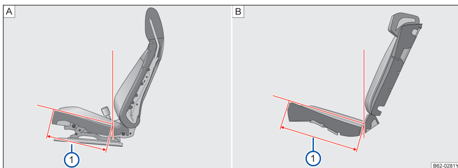
图 63 座椅坐垫深
