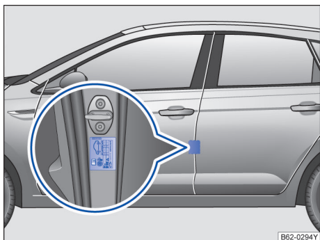
图 154 驾驶员侧中间门柱上：胎压标签（或者在油箱盖的内侧）
