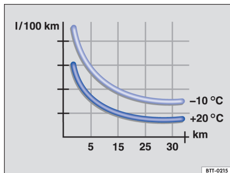
图 86 两种不同环境温度时的百公里油耗
