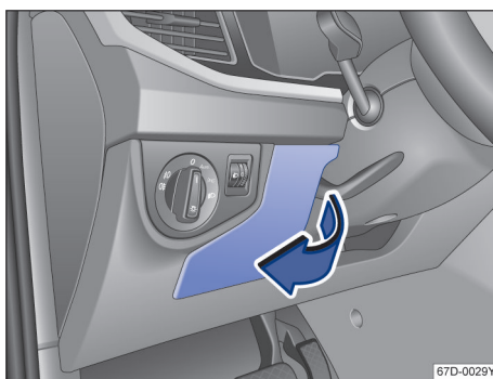
图 132 保险丝盒盖板
