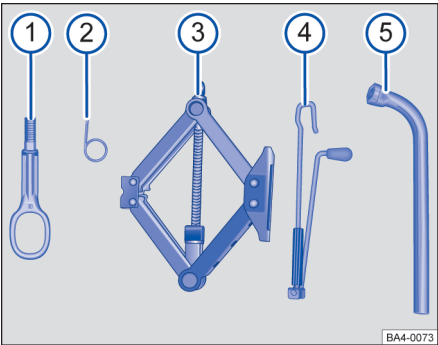
图 128 随车工具的组件
