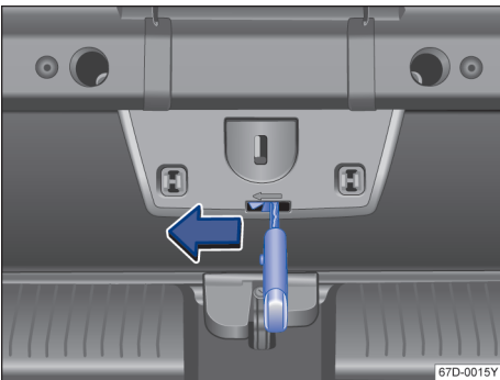
图 55 在行李厢中：行李厢盖的应急解锁机构
