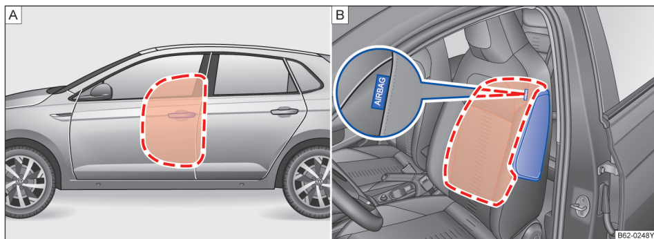
图 34 [A]: 汽车左侧 - 侧面安全气囊膨胀范围; [B]: 左前座椅侧面 - 侧面安全气囊安装位置及膨胀范围
