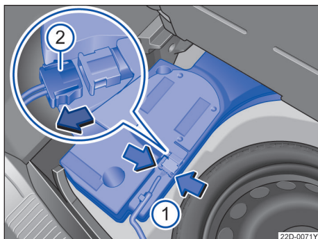
图 158 行李厢内：拆下重低音扬声器
