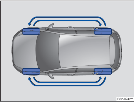
图 150 前后车轮换位
