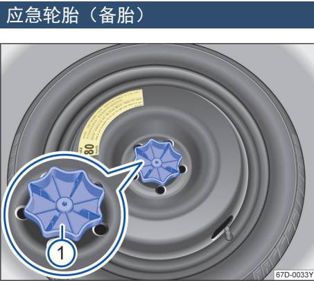
图 151 行李厢内：备用车轮固定手轮
